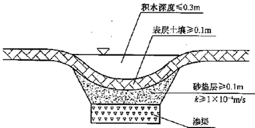
图 12 浅沟—渗渠组合
