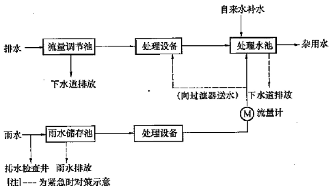
图 2 雨水、中水结合的工艺流程图
