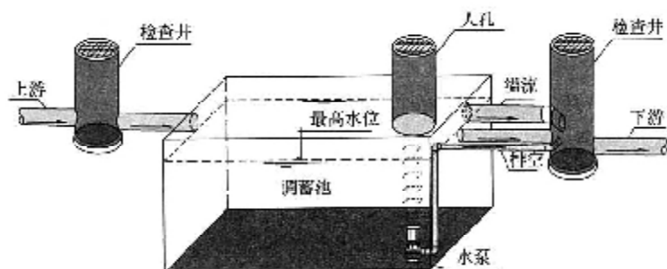
图 23 调蓄池示意
