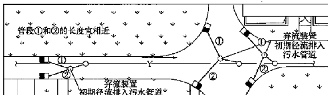
图 6 地面雨水收集弃流装置布置
