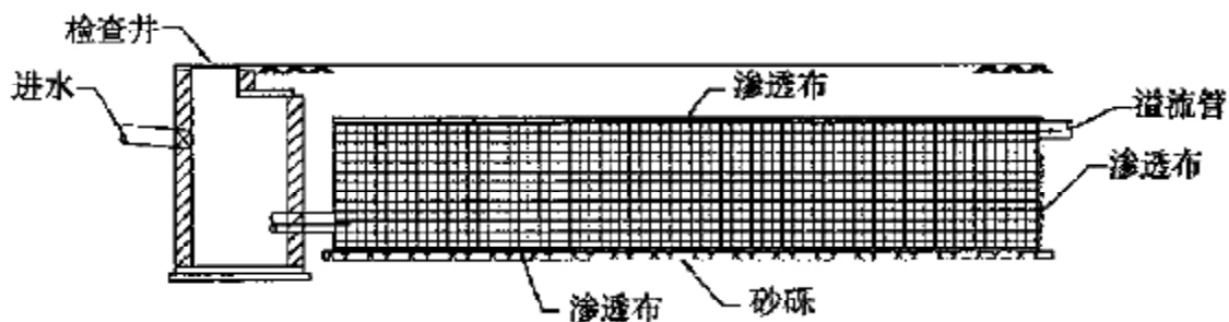
图 14 塑料模块拼装组合式水池
