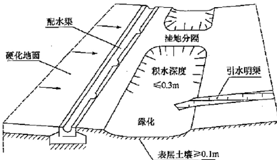
图 11 洼地入渗系统
