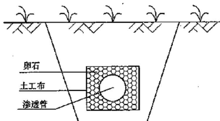
图 13 渗透管沟断面
