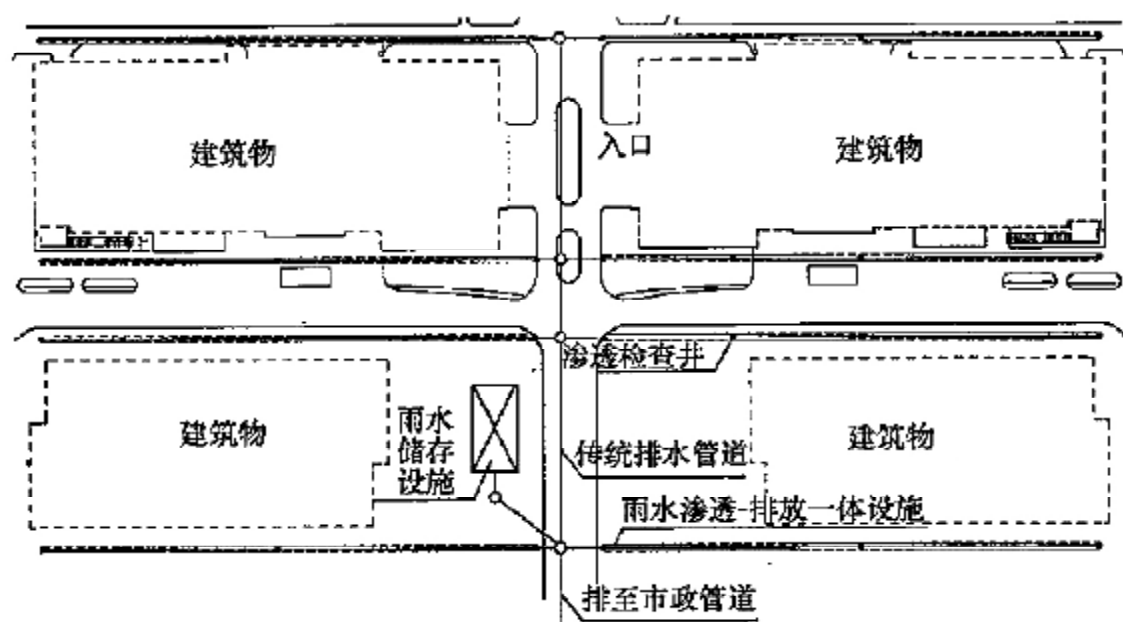
图 8 局部场所渗排一体
