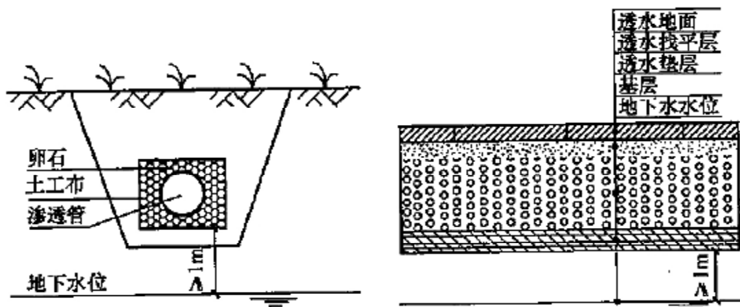
图 1 入渗面距地下水位应大于 1m
