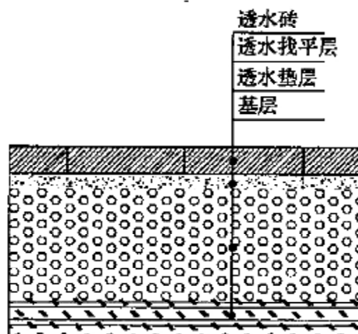
图 10 透水铺装地面结构示意图
