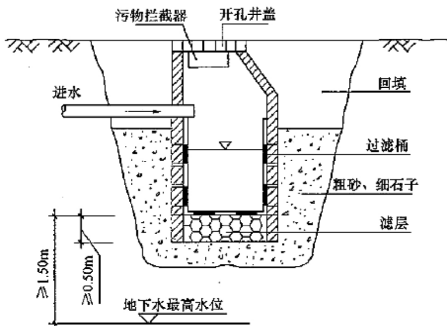
图 15 渗井 A
