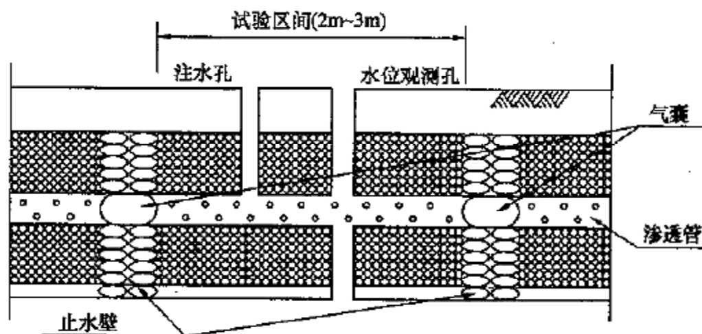
图 24 渗透管沟试验段设置示意
