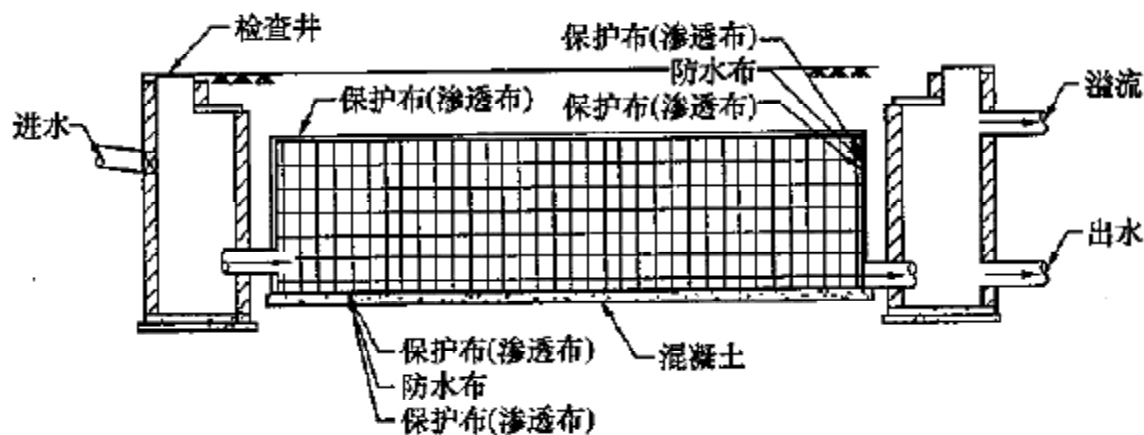
图 20 塑料模块蓄水池
