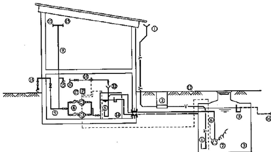
图 19 雨水蓄存利用系统示意
