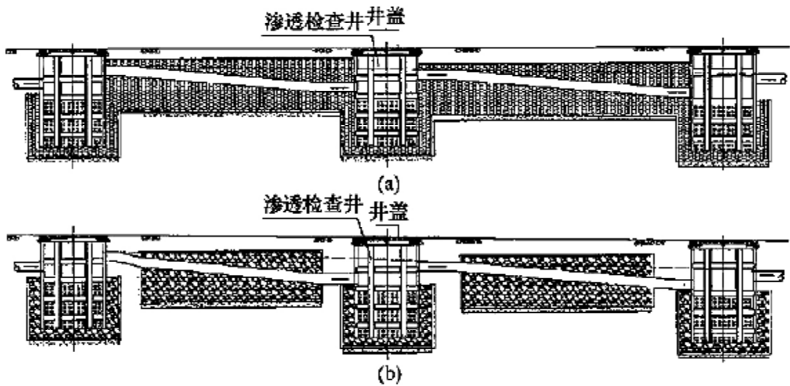
图9 渗透(管)-排水一体设施构造断面
