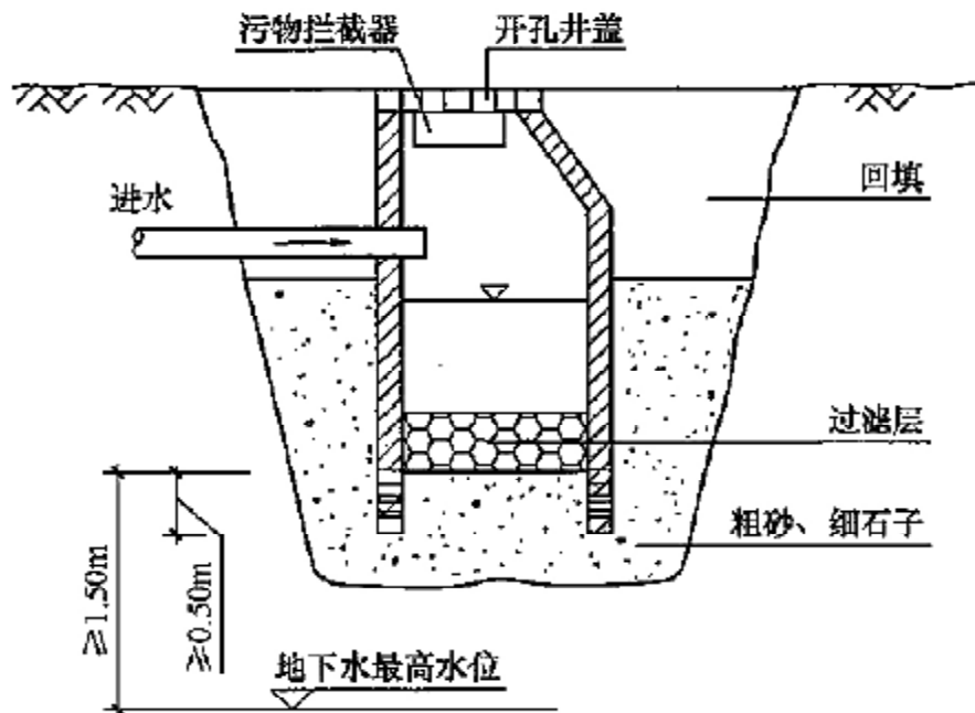
图 16 渗井 B
