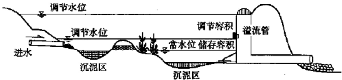
图 22 湿塘
